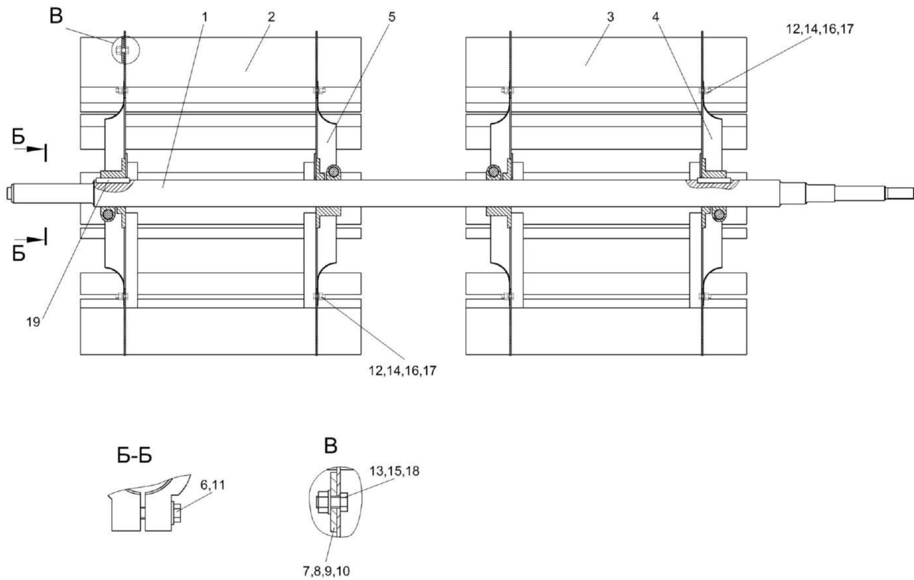
Рисунок 60 – Крылач КЗК-10-0217010
