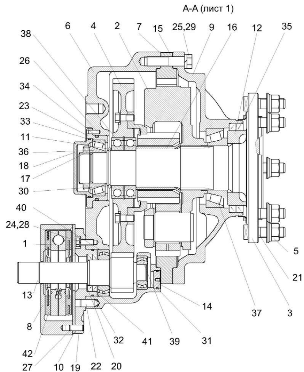
Рисунок 43 – Редуктор КЗК-12-0107190 (лист 2)
