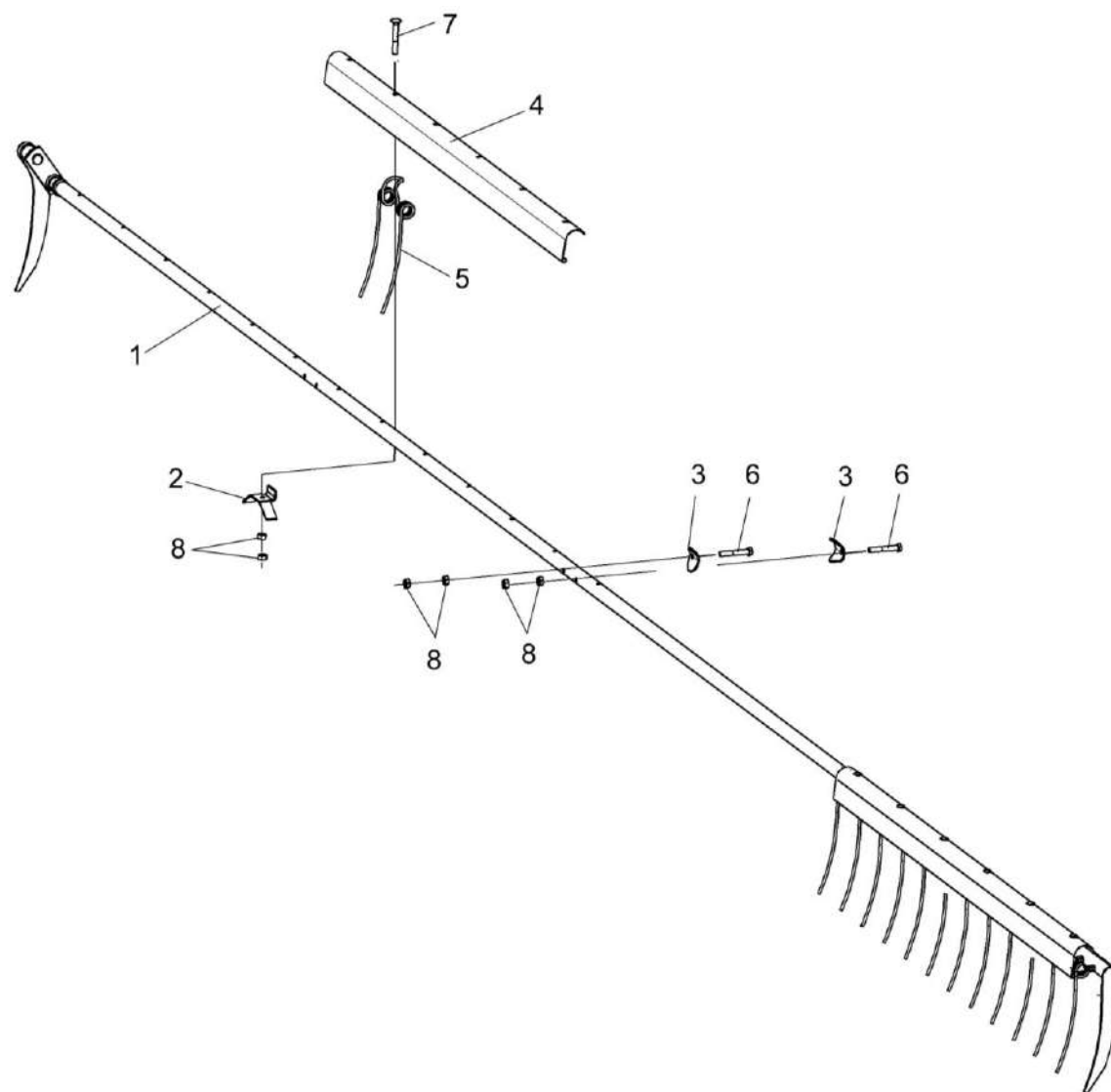
Рисунок 283 – Граблина КЗР 1373550
