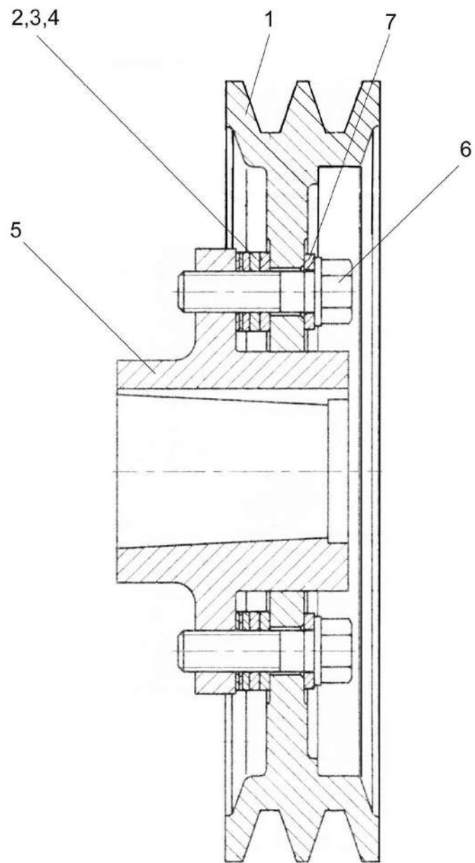
Рисунок 178 – Шкив K3K 0290090
