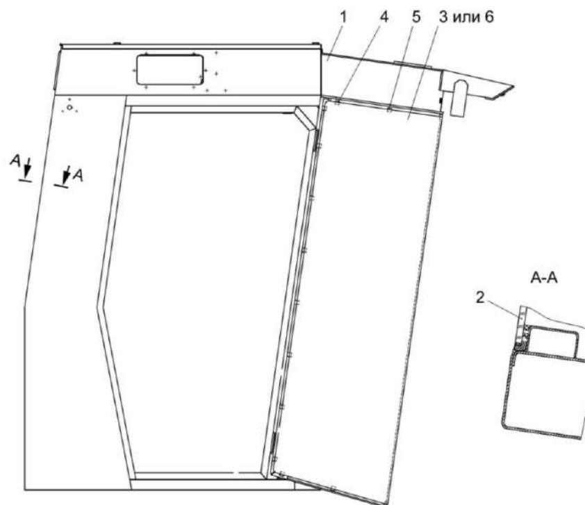
Рисунок 246 – Каркас КЗК-10-0120010А
