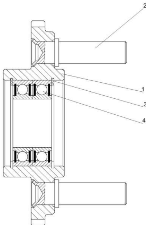
Рисунок 71 – Колесо КЗК-12-0202720
