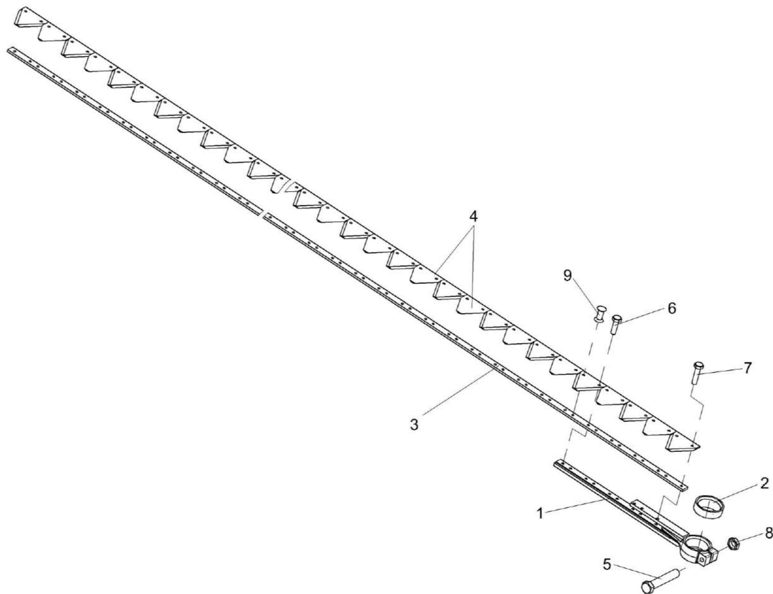
Рисунок 267 – Нож КЗР 1507010-21
