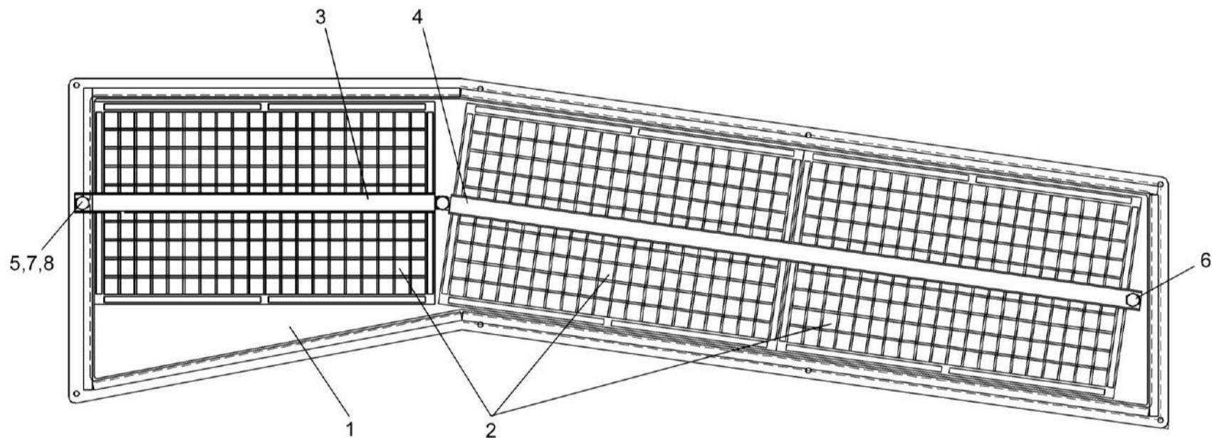
Рисунок 249 – Фильтр СЭУ 0201140-01
