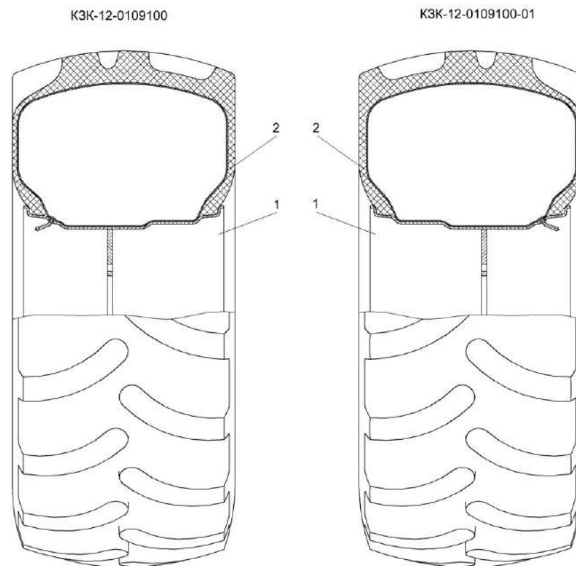
Рисунок 57 – Колеса КЗК-12-0109100, КЗК-12-0109100-01
