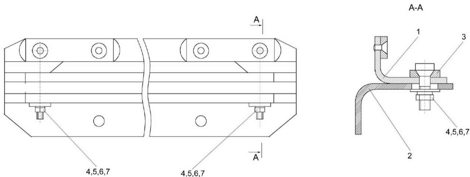
Рисунок 223 – Успокоитель КЗК 1870160
