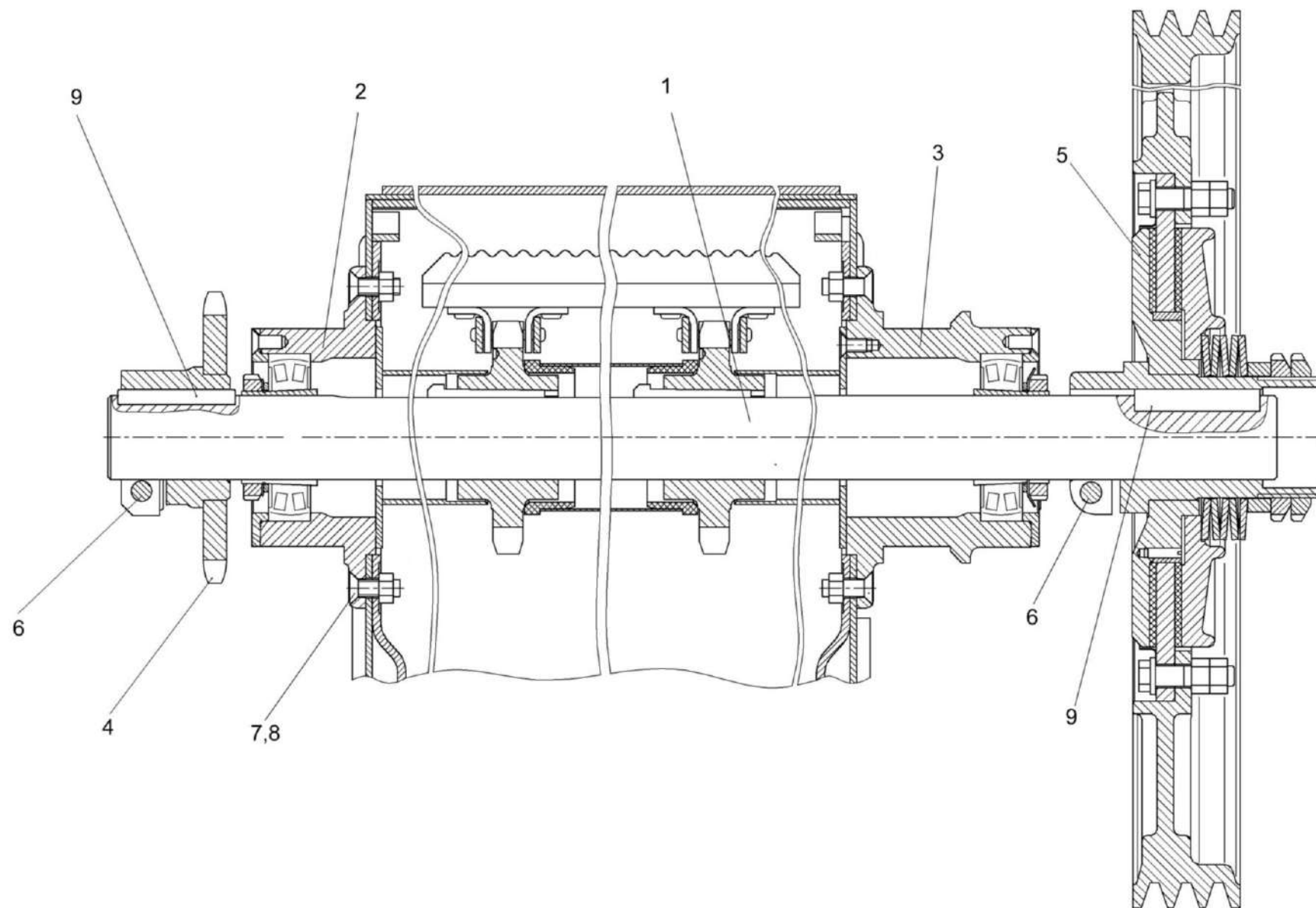
Рисунок 208 – Установка вала верхнего K3K-12-1803000A
