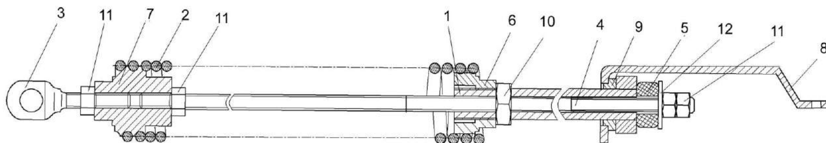
Рисунок 233 – Пружина КЗР-10-0100580
