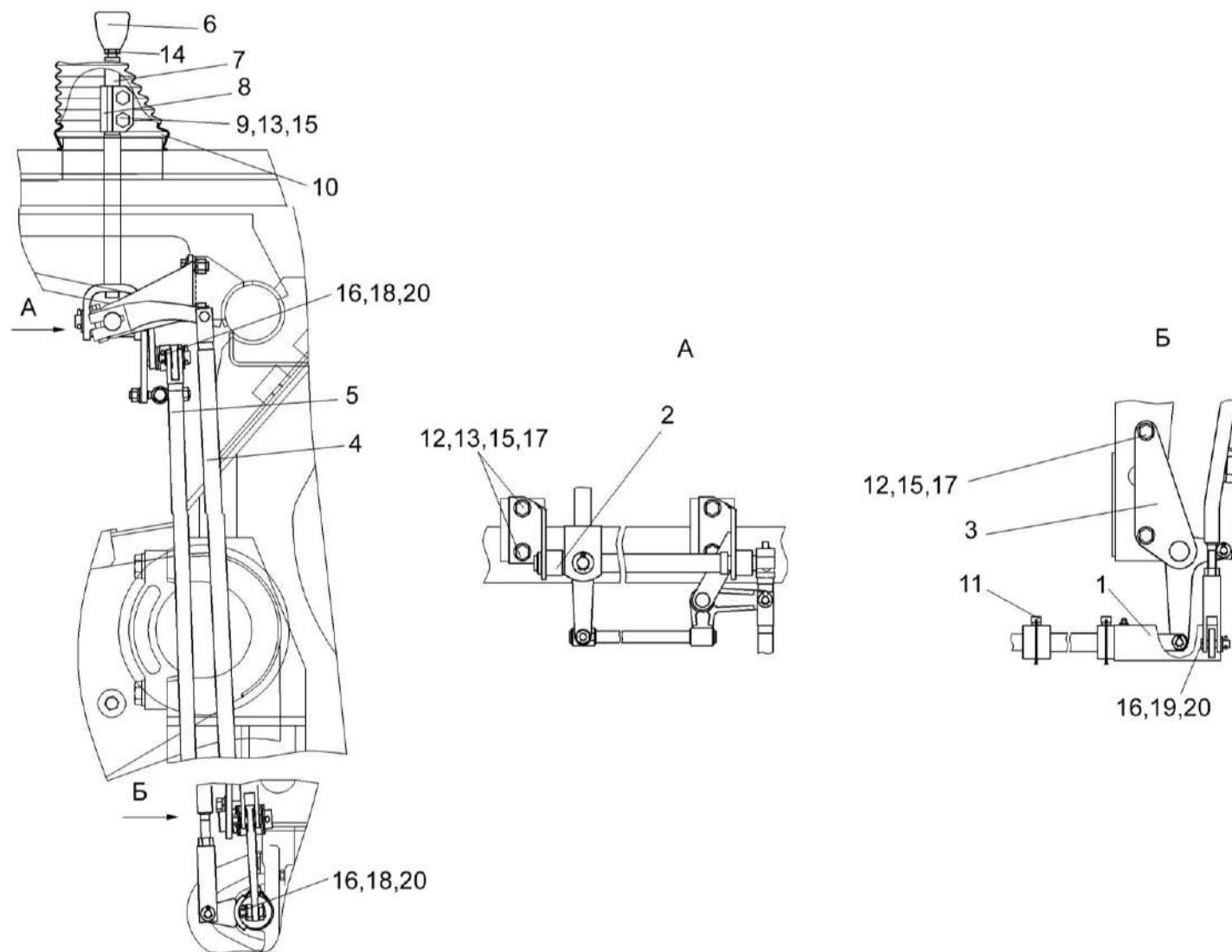
Рисунок 136 – Механизм управления коробкой диапазонов КЗК-12-0119040А
