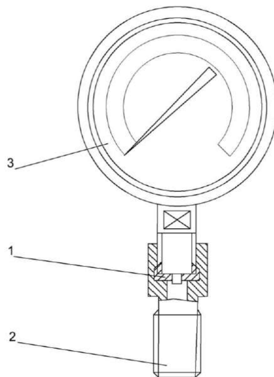
Рисунок 200 – Манометр УЭС-7-0602810
