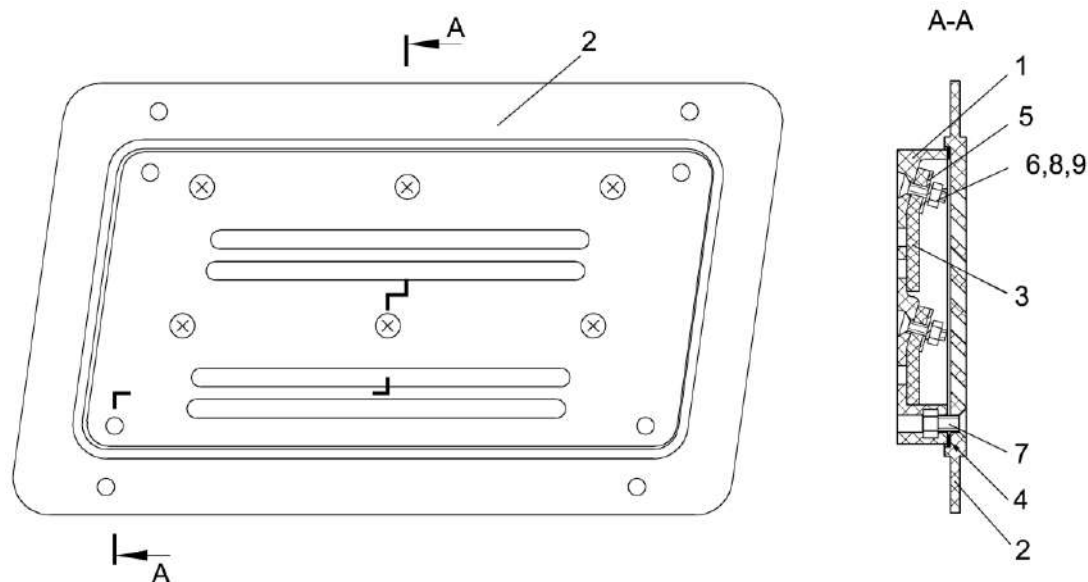
Рисунок 248 – Клапан СЭУ 0200610
