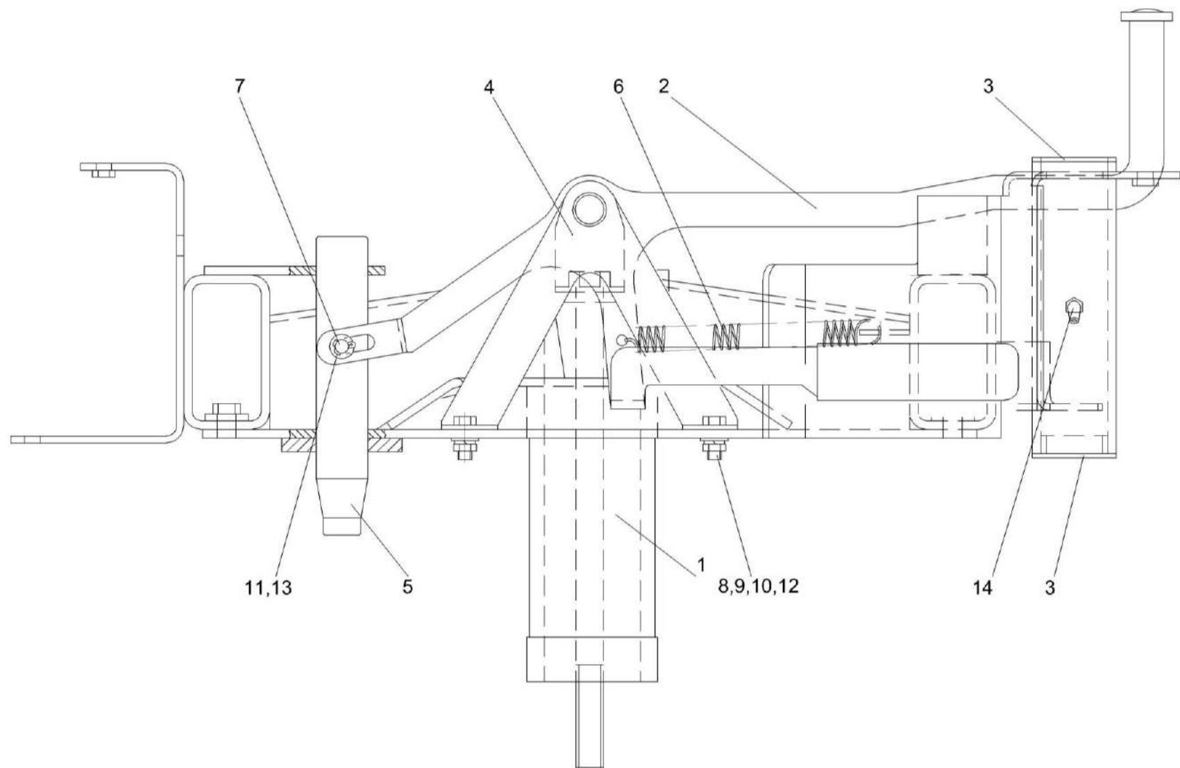
Рисунок 117 – Рама K3K-12-0117010 A
