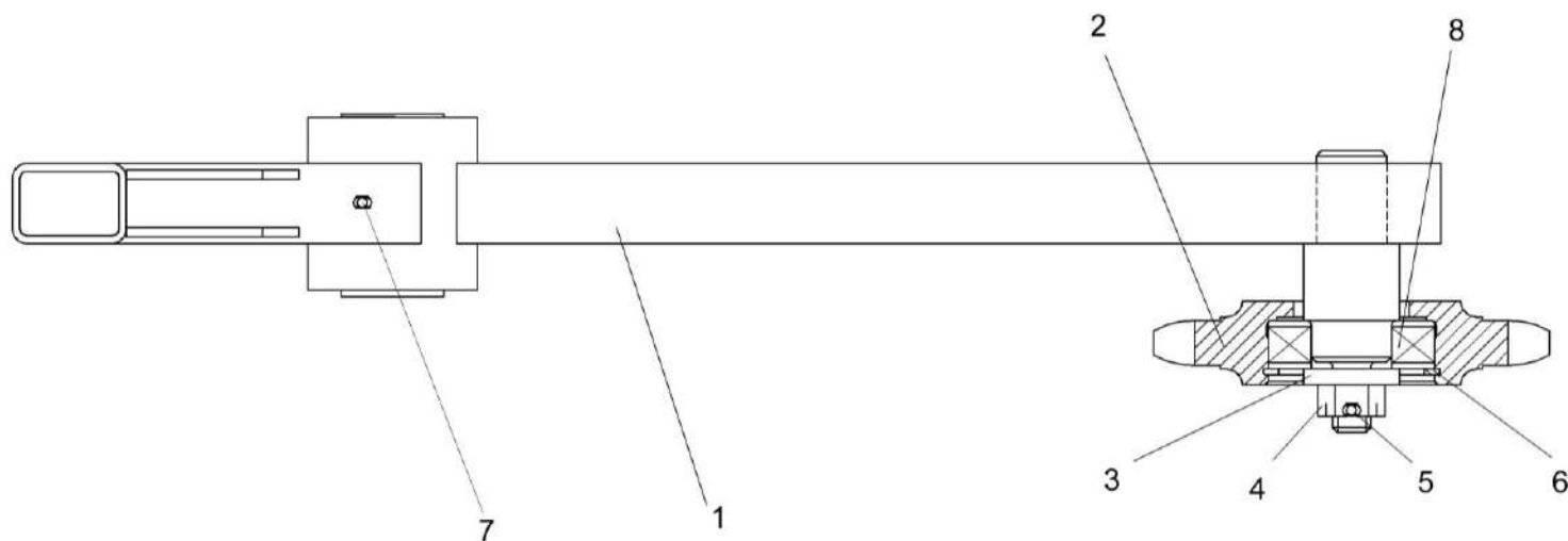
Рисунок 236 – Рычаг КЗР-10-0100680А
