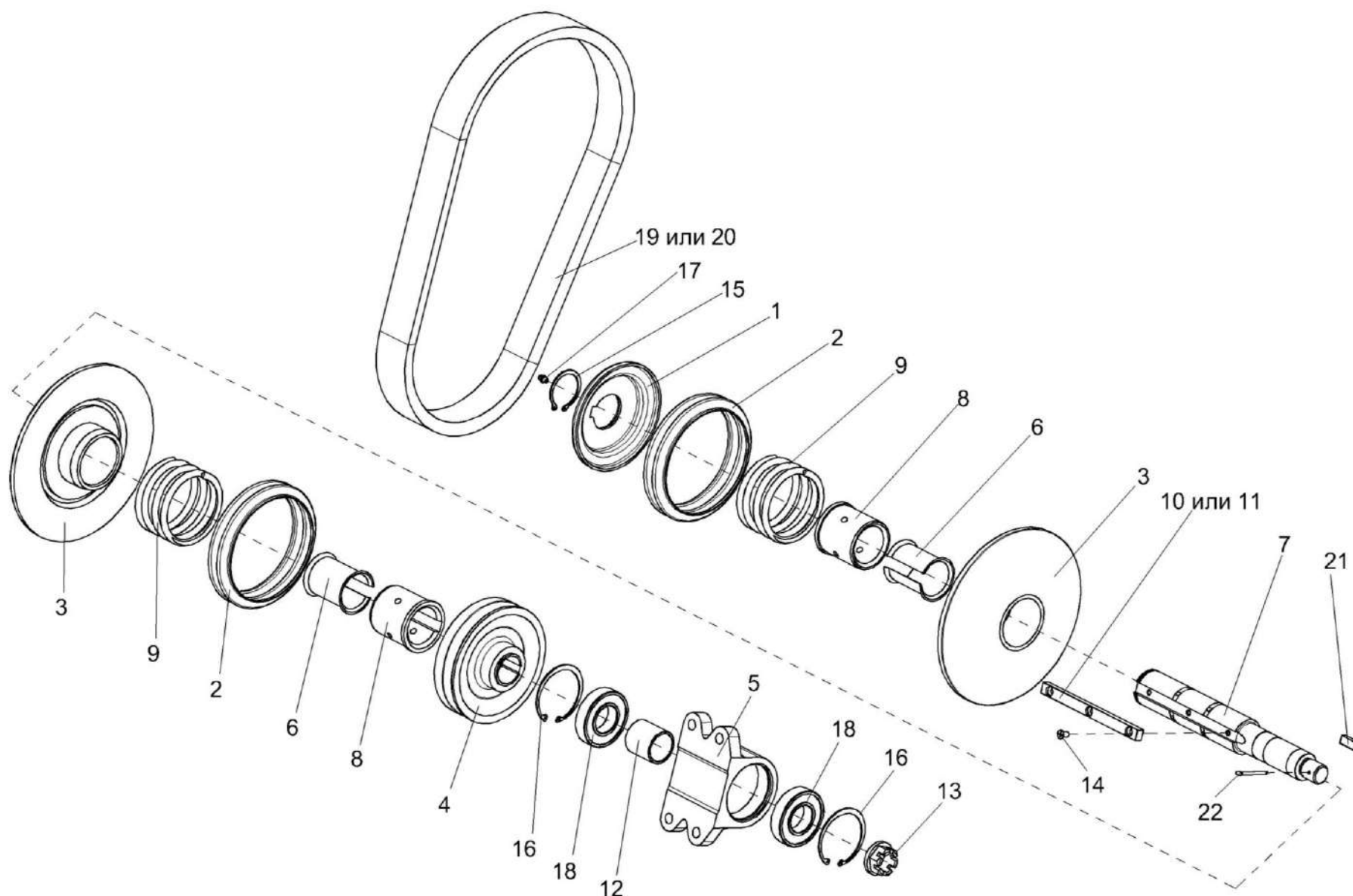
Рисунок 270 – Вариатор КЗР 1514200
