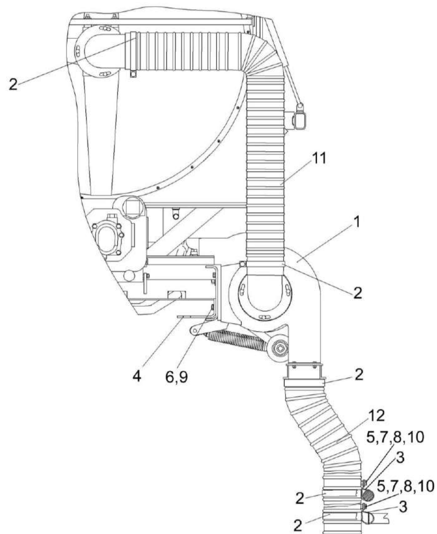
Рисунок 238 – Установка вентилятора K3K-10-0112240
