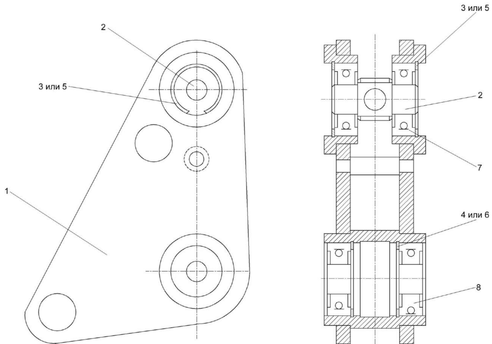
Рисунок 219 – Рычаг КЗК-12-1808500
