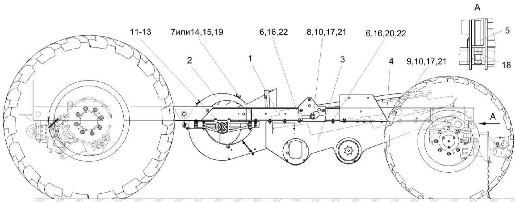
Рисунок 39 – Шасси КЗК-12-0111000А (вид сбоку)
