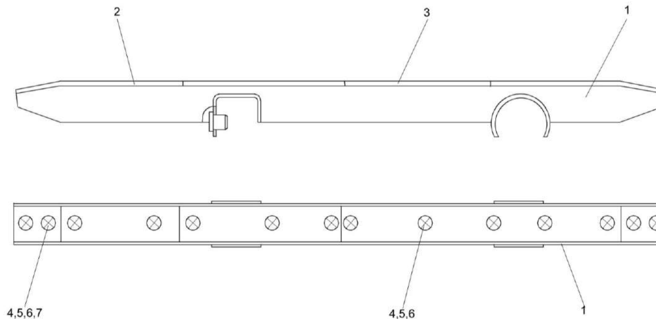
Рисунок 206 – Успокоитель КЗК 1770050
