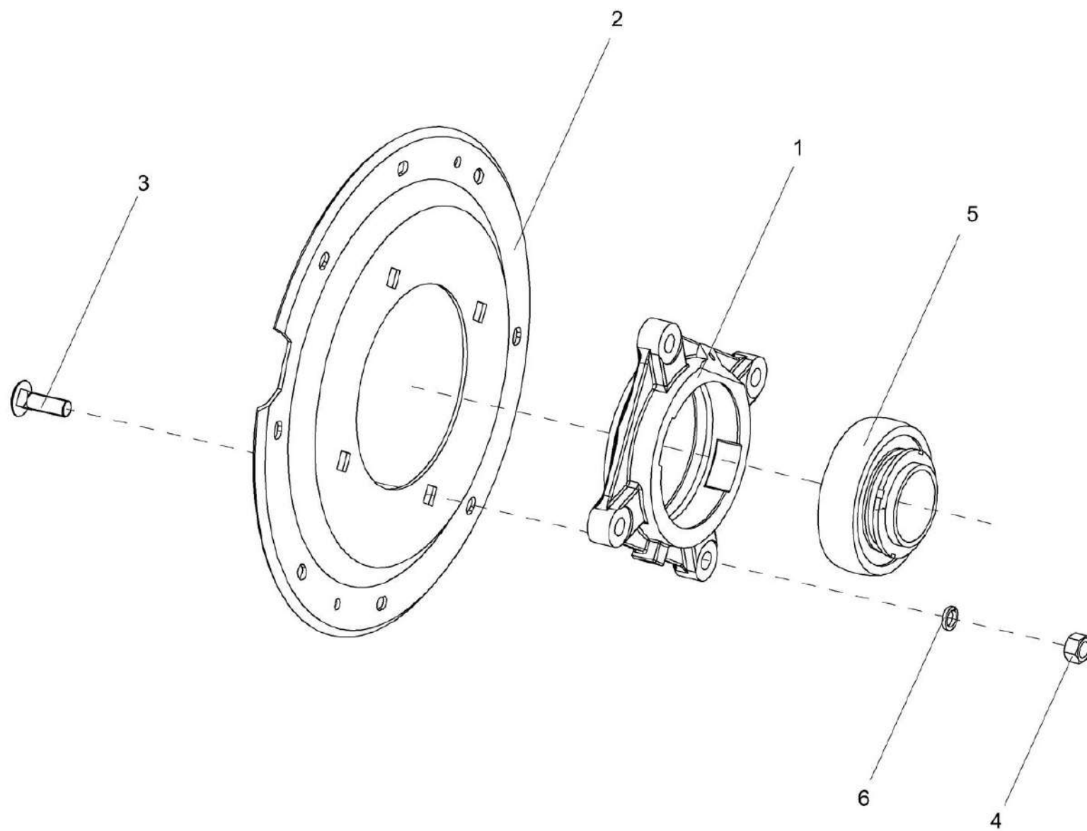
Рисунок 30 – Фланец КЗК-10-0102070
