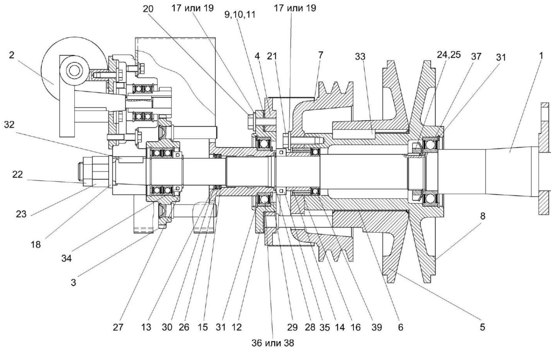
Рисунок 69 – Контрпривод вариатора K3K-12-0202500
