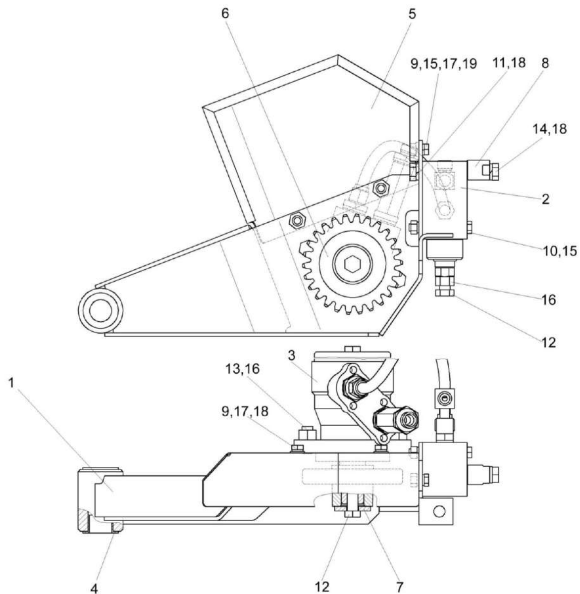
Рисунок 226 – Гидрореверс КЗК-12-1804000А
