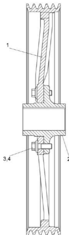
Рисунок 72 – Шкив КЗК-12-0202860А
