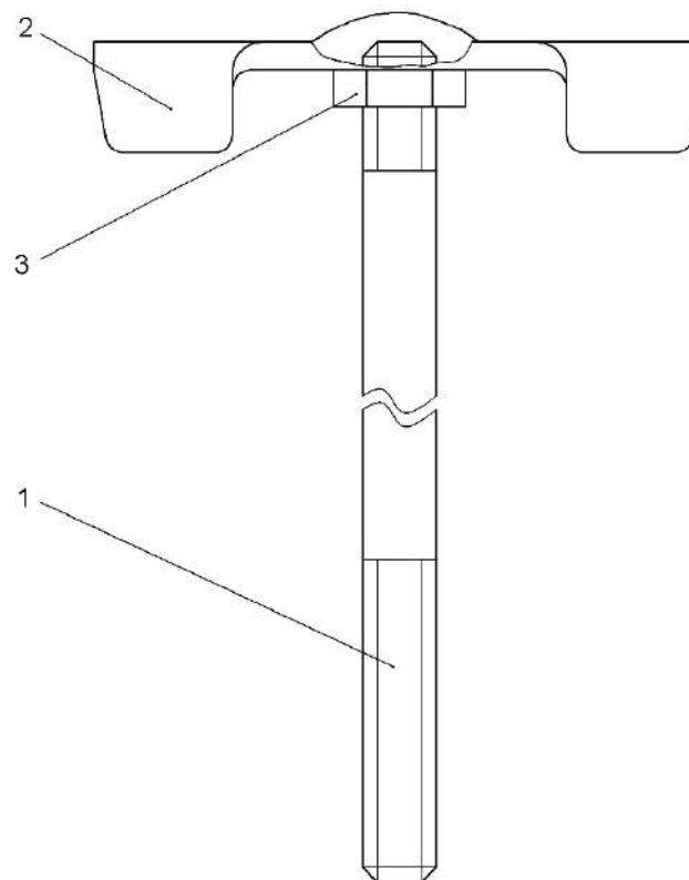
Рисунок 134 – Зажим УЭС 0302540
