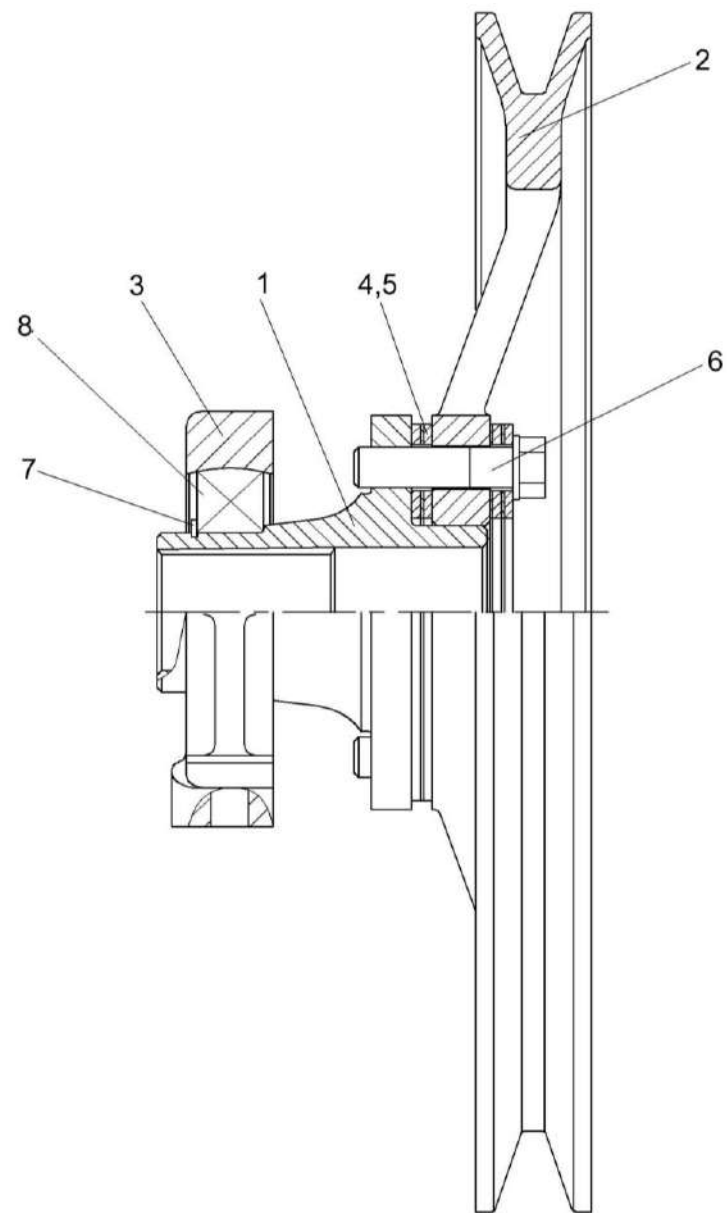
Рисунок 75 – Шкив КЗК-10-0212060
