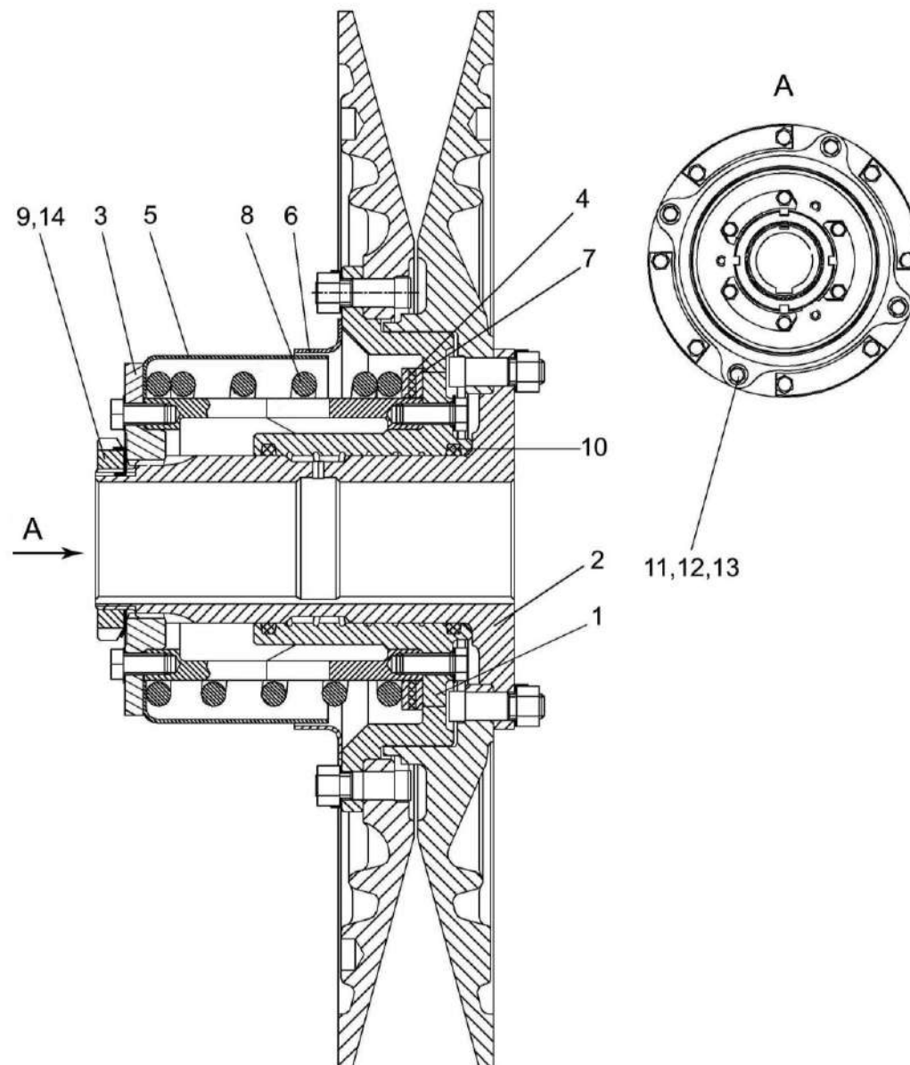
Рисунок 33 – Вариатор барабана K3K 0123000
