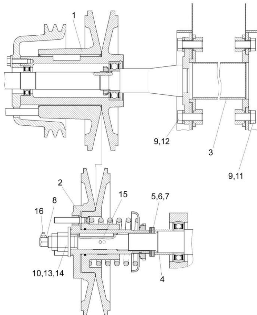
Рисунок 22 – Установка котрпривода вариатора K3K-12-0202500
