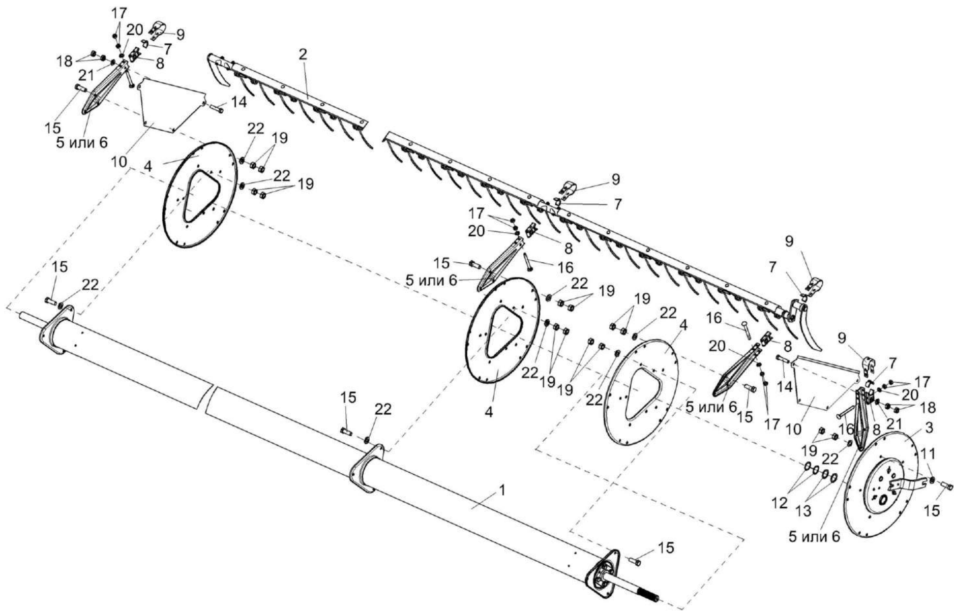
Рисунок 282 – Мотовило КЗР 1573500
