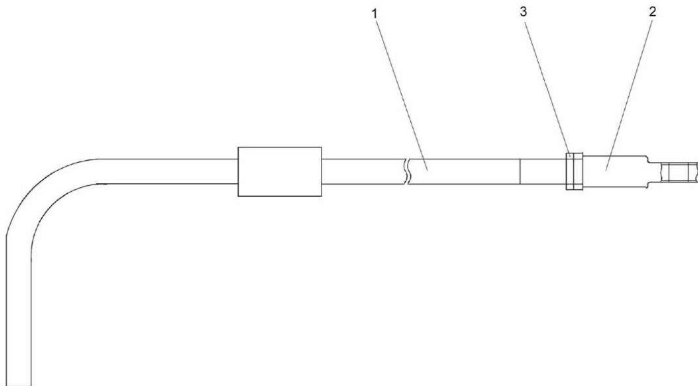
Рисунок 221 – Тяга КЗК 1780020
