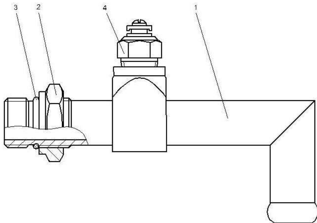
Рисунок 184 – Тройник КЗК-12-601300
