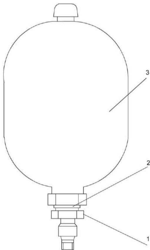
Рисунок 198 – Пневмогидроаккумулятор УЭС-7-0602440
