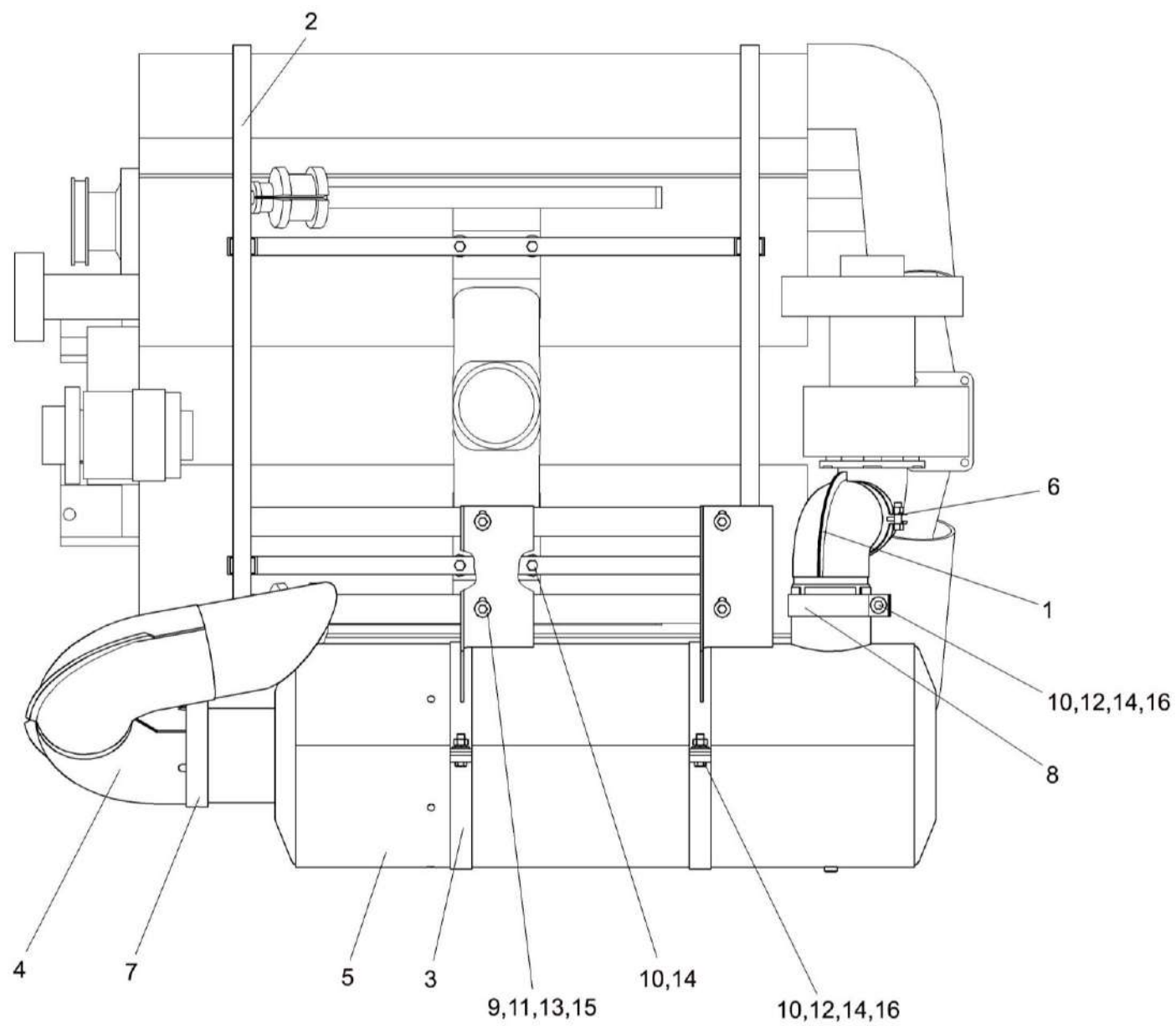
Рисунок 102 – Установка глушителя КЗК-12-0106170
