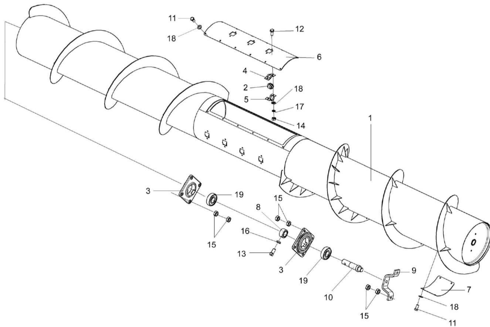
Рисунок 265 – Шнек КЗР 1502140-21
