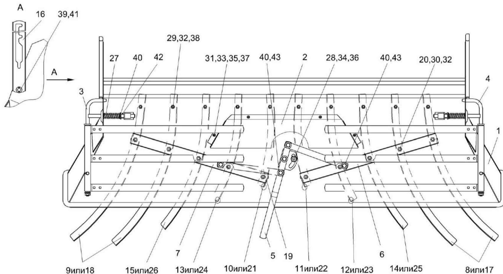
Рисунок 179 – Дефлектор КЗК-12-0290020
