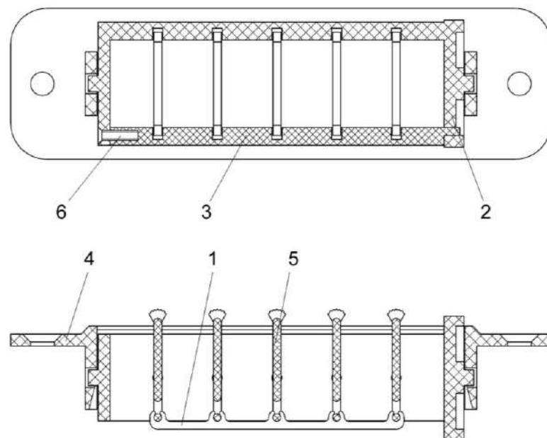
Рисунок 250 – Дефлектор СЭУ 0200690-01
