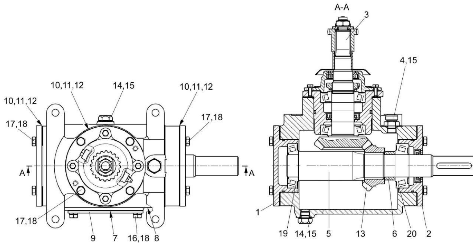
Рисунок 162 – Редуктор КЗК-12-0209000
